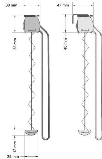
Top Fix
